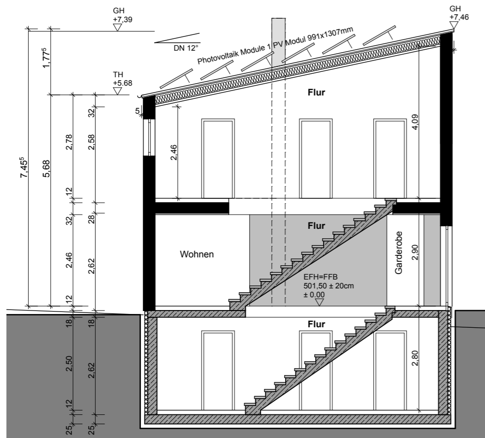
SCHNITT
