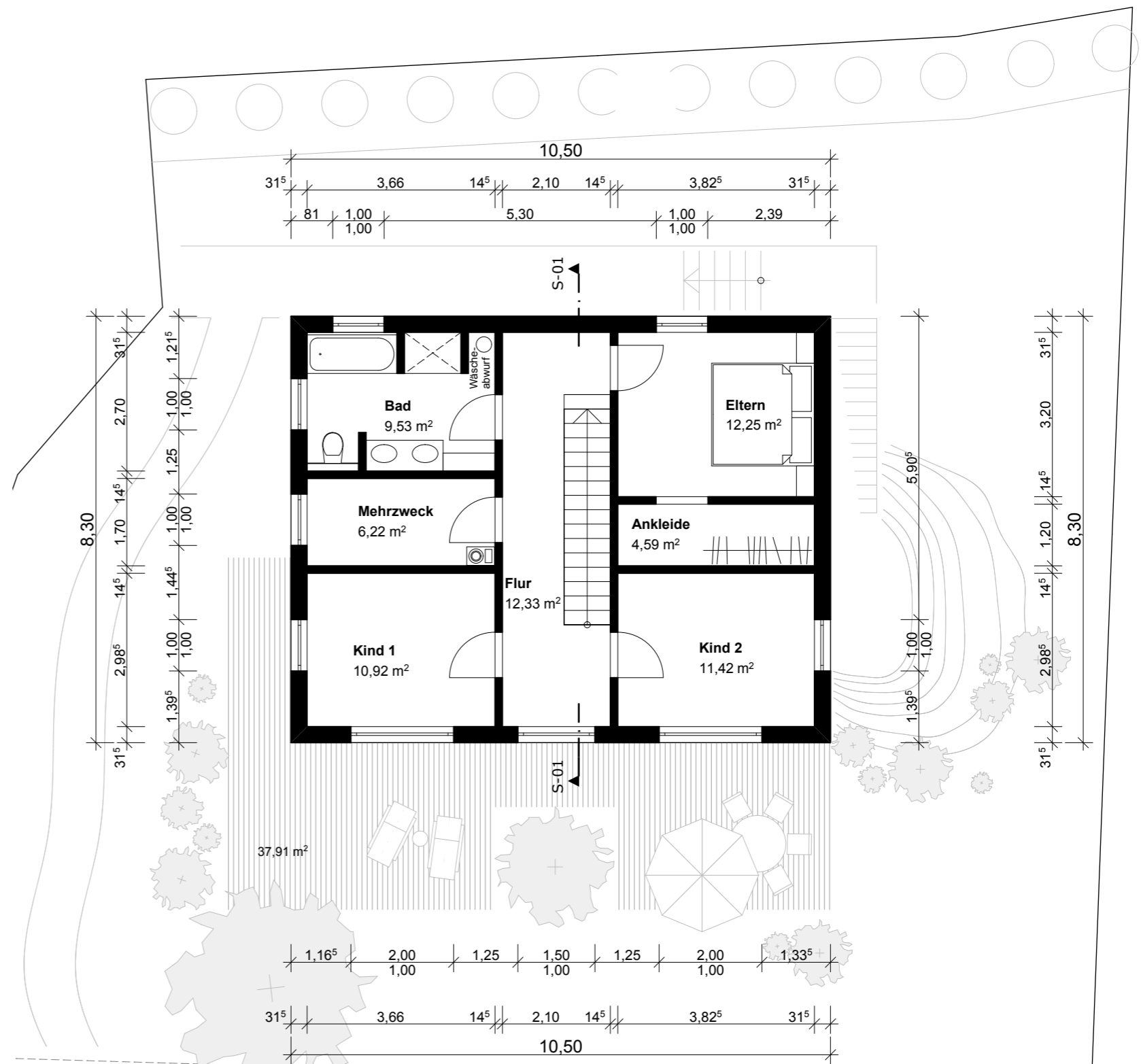
OBERGESCHOSS
