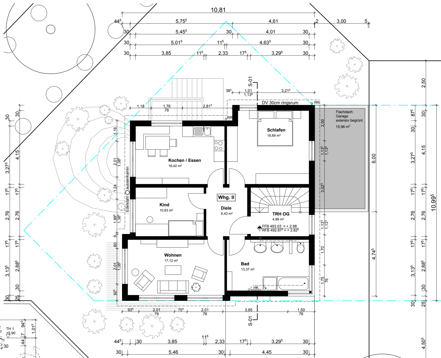
OBERGESCHOSS
