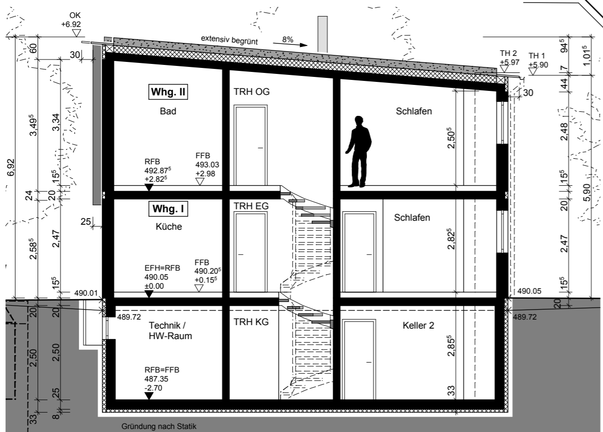
SCHNITT
