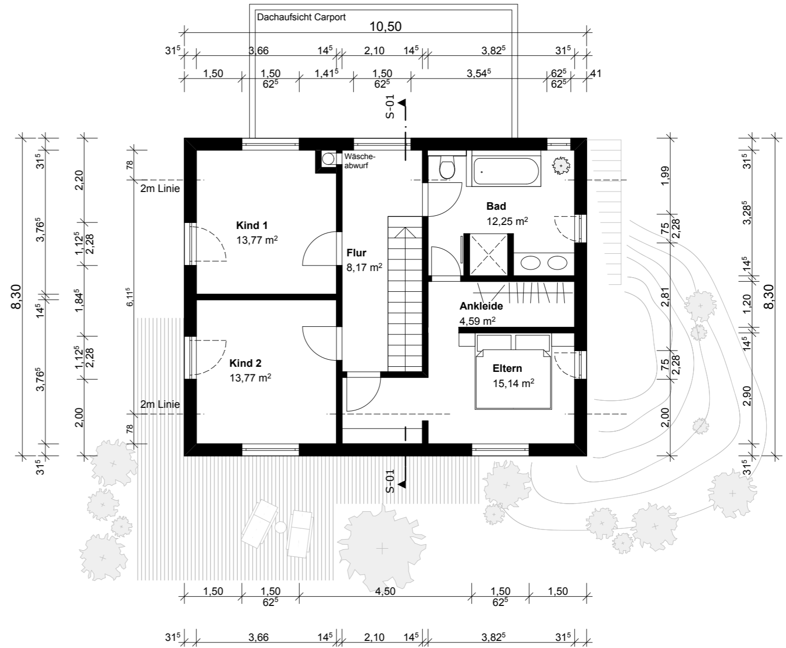
OBERGESCHOSS
