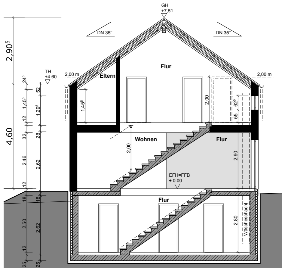
SCHNITT
