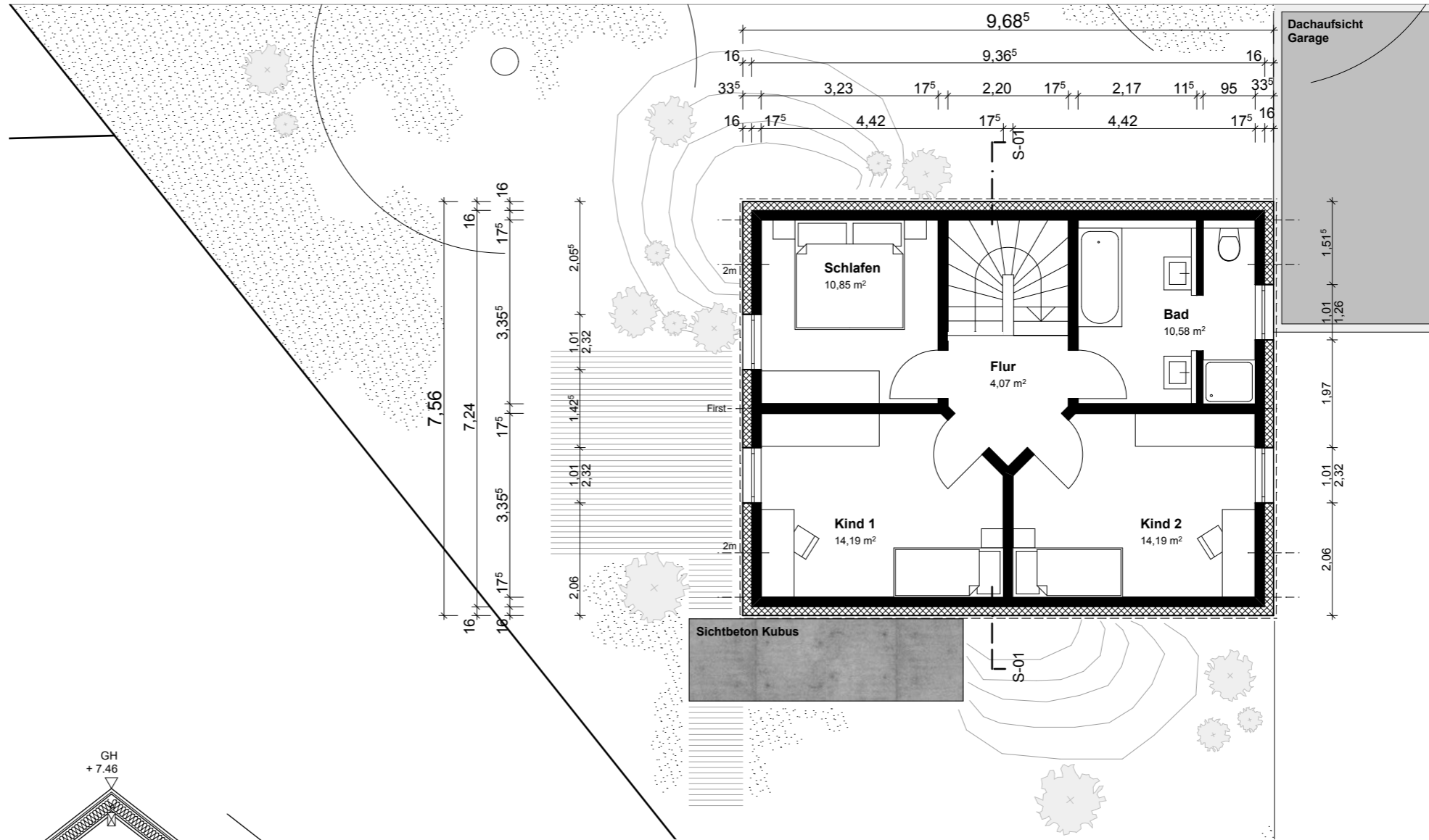
OBERGESCHOSS
