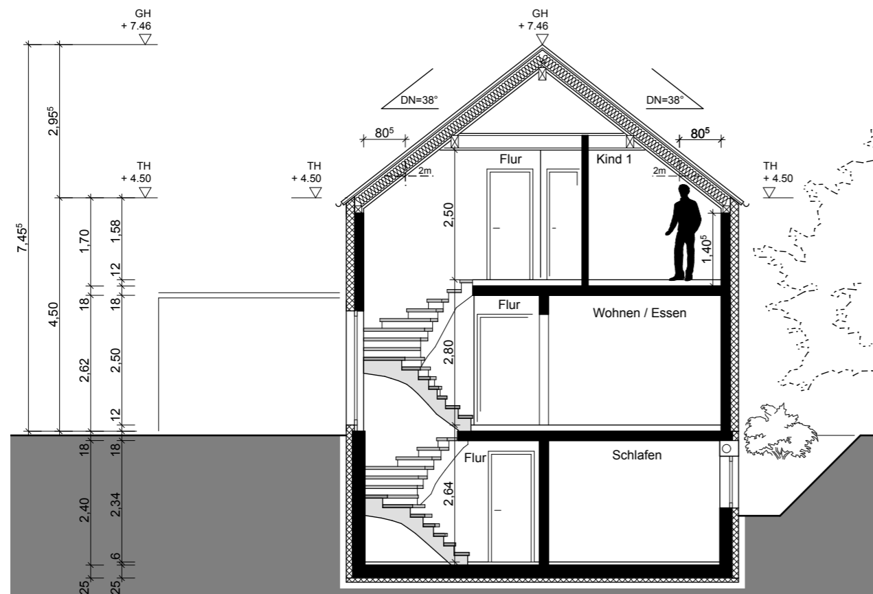
SCHNITT
