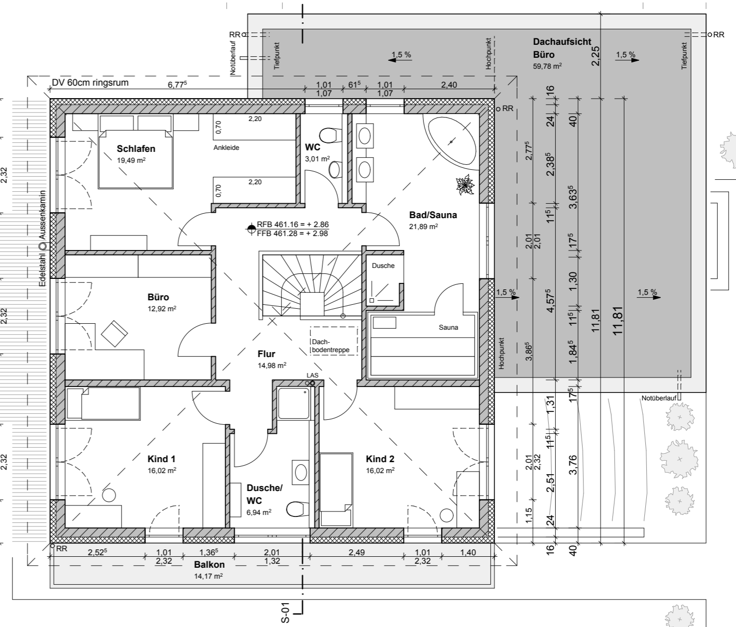
OBERGESCHOSS
