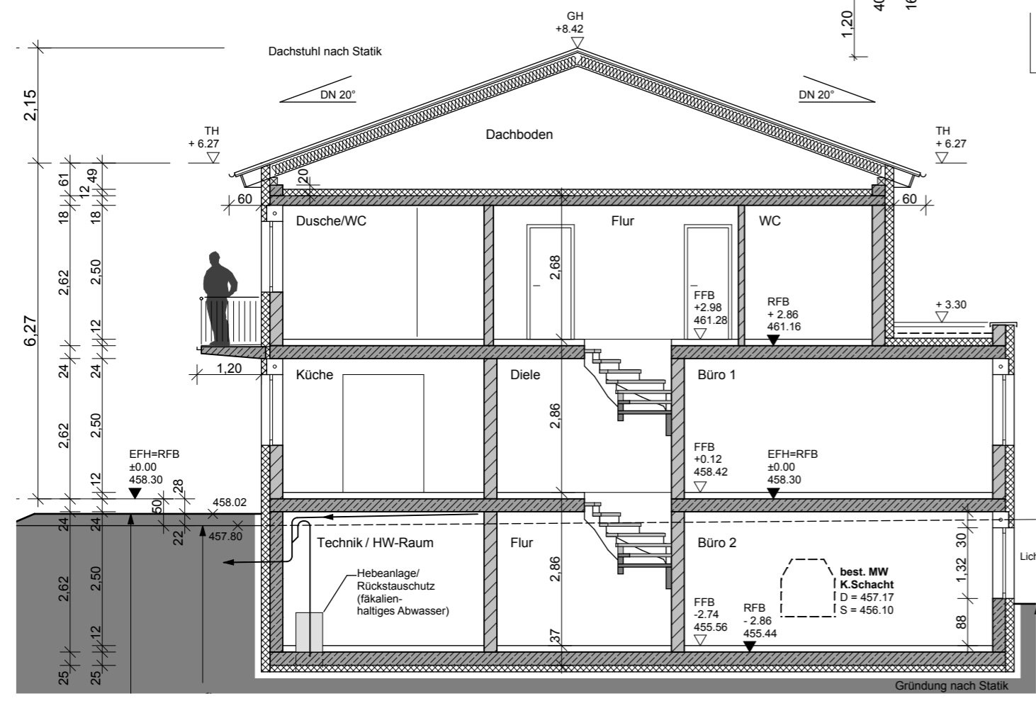
SCHNITT
