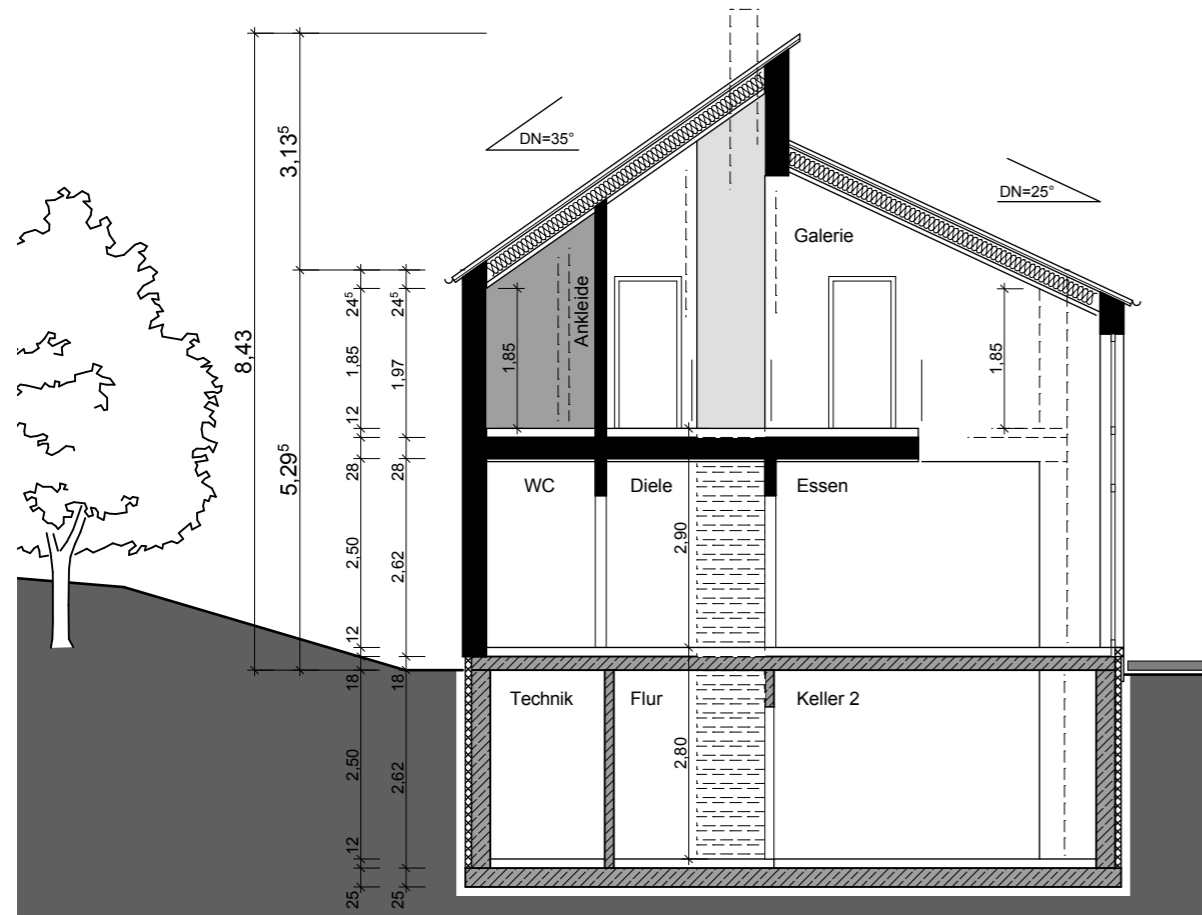
SCHNITT
